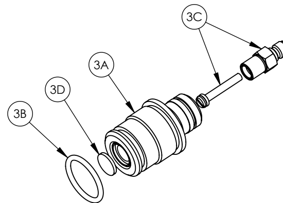
ITEM 3, FILL ADAPTER
